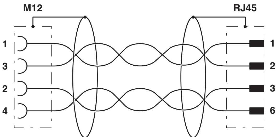
Przyporządkowanie styków gniazda M12 i wtyku RJ45
