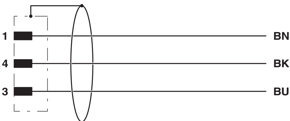
Schemat
