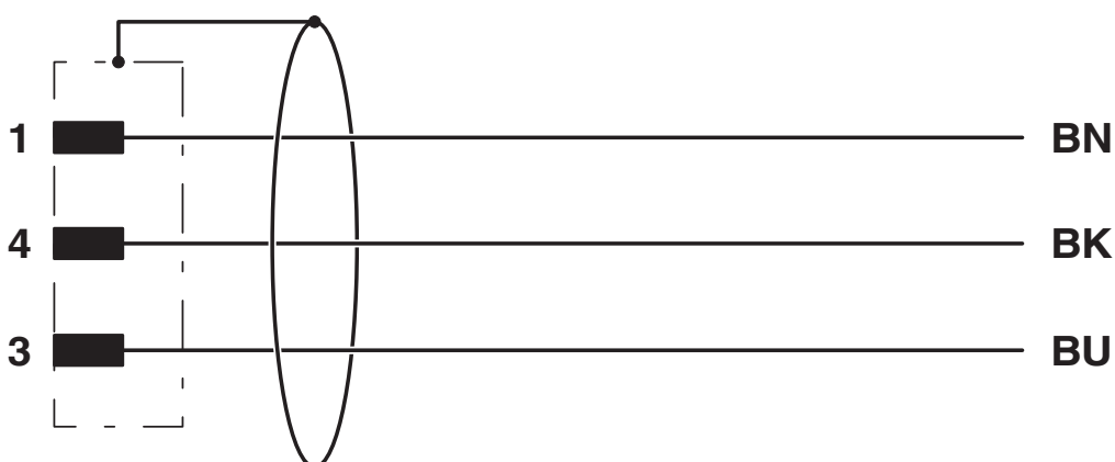
Schemat
