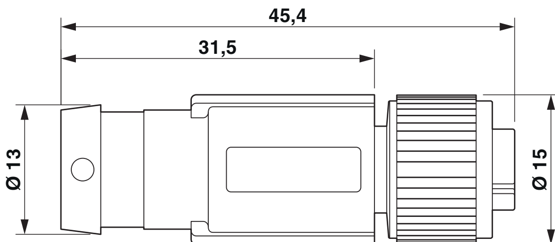
Wtyk z gniazdem M12 x 1, prosty, ekranowany
