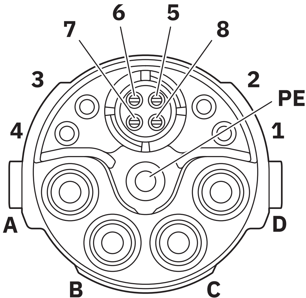
Układ styków gniazda CAT5
