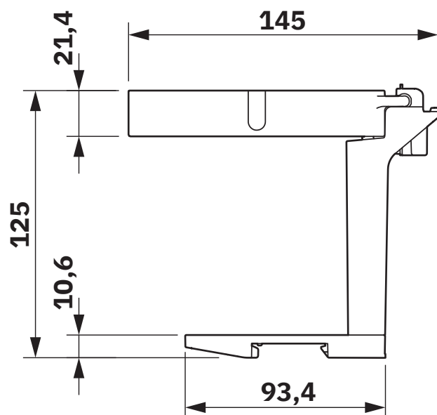
Rysunek wymiarowy
