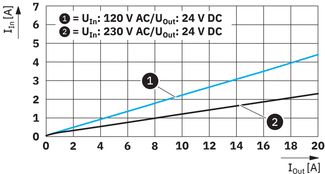
Prąd wejściowy/wyjściowy
