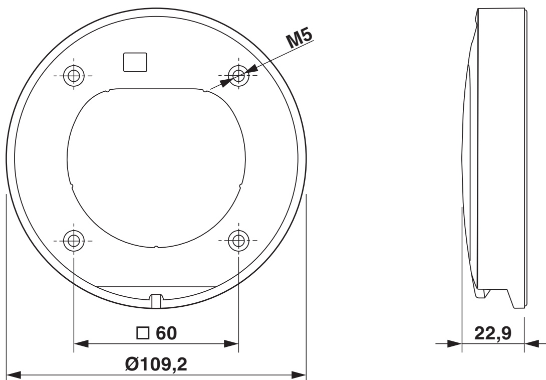
Rysunek wymiarowy
