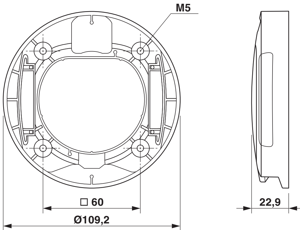
Rysunek wymiarowy
