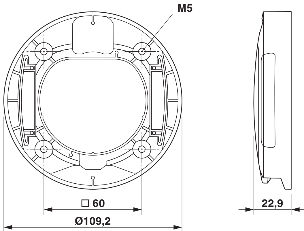
Rysunek wymiarowy
