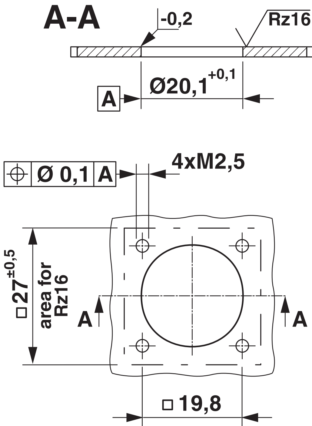
Rysunek wymiarowy
