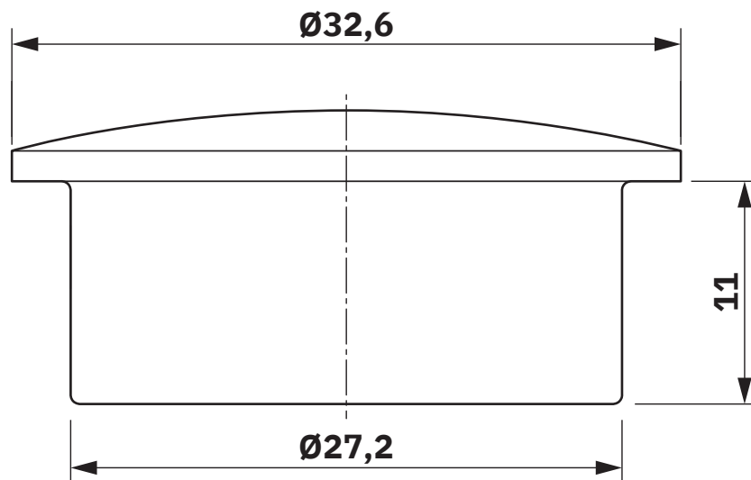
Rysunek wymiarowy
