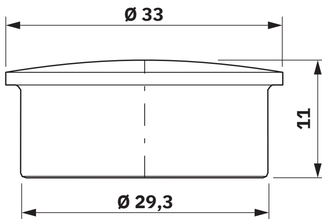
Rysunek wymiarowy
