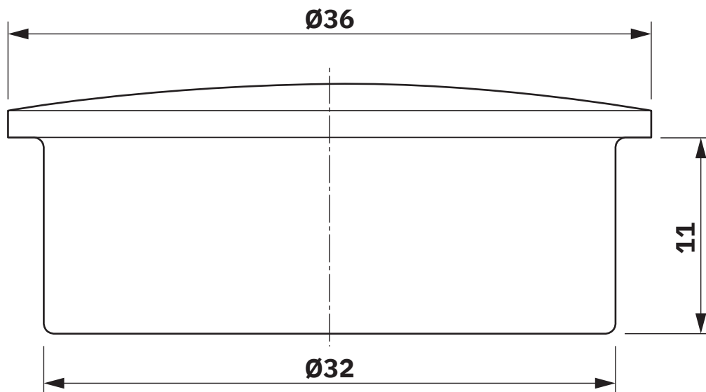
Rysunek wymiarowy
