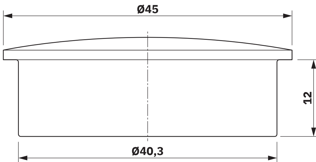
Rysunek wymiarowy
