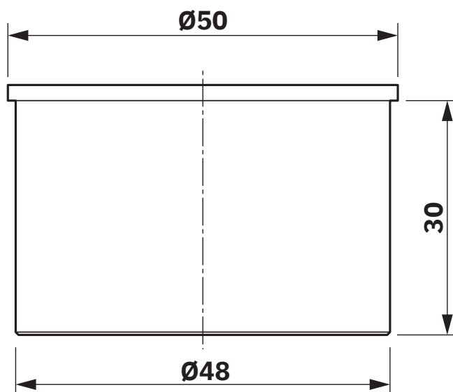
Rysunek wymiarowy
