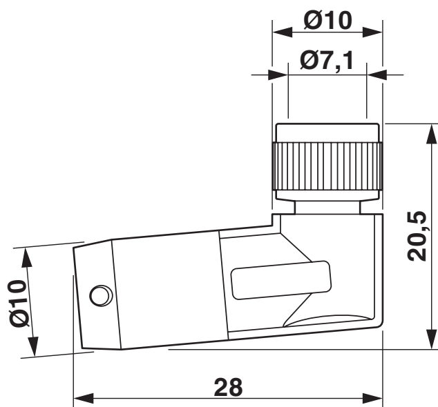
Rysunek wymiarowy
