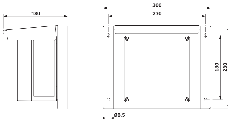
Rysunek wymiarowy
