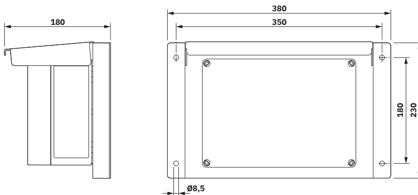
Rysunek wymiarowy
