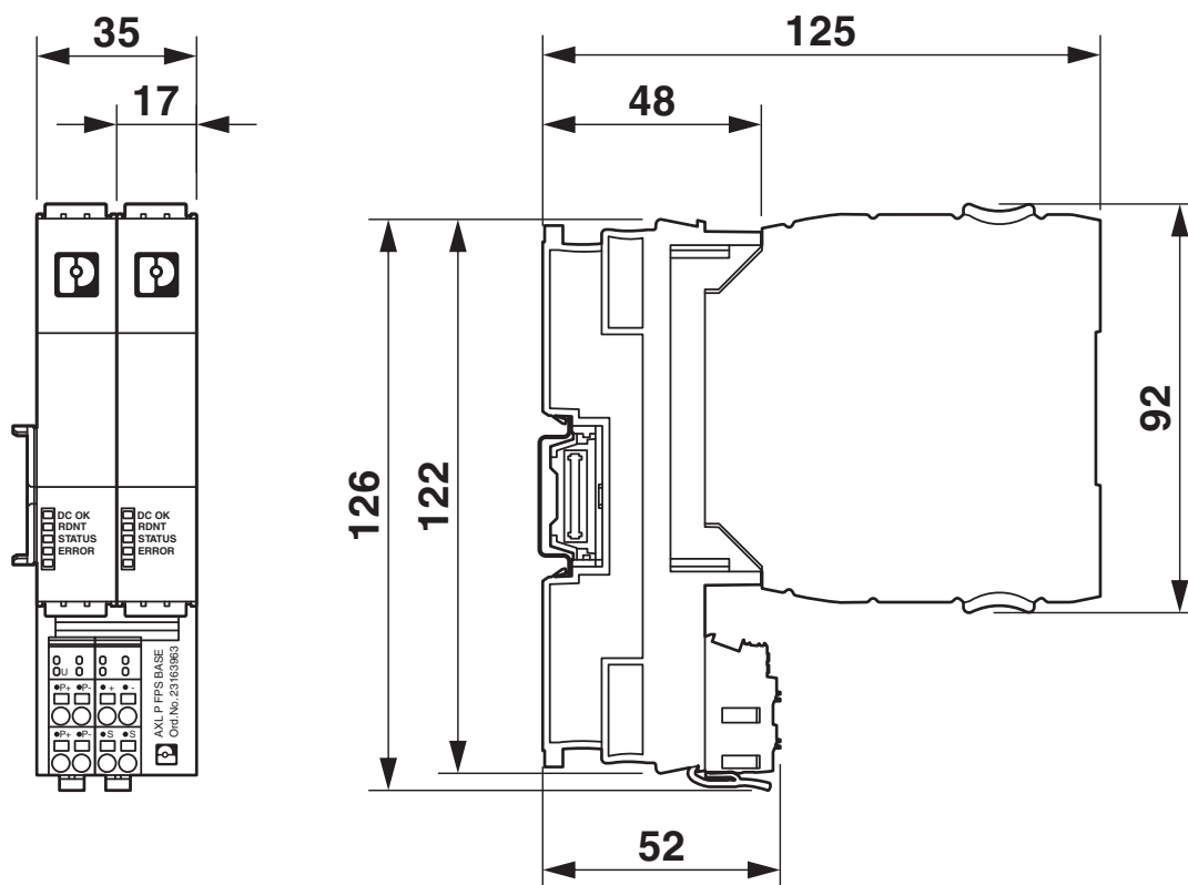
Rysunek wymiarowy
