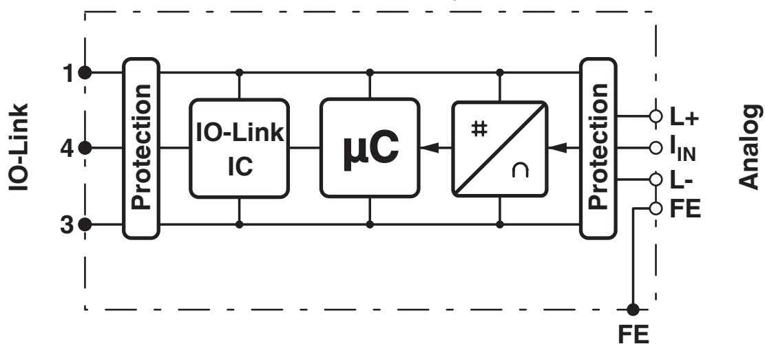
Schemat blokowy
