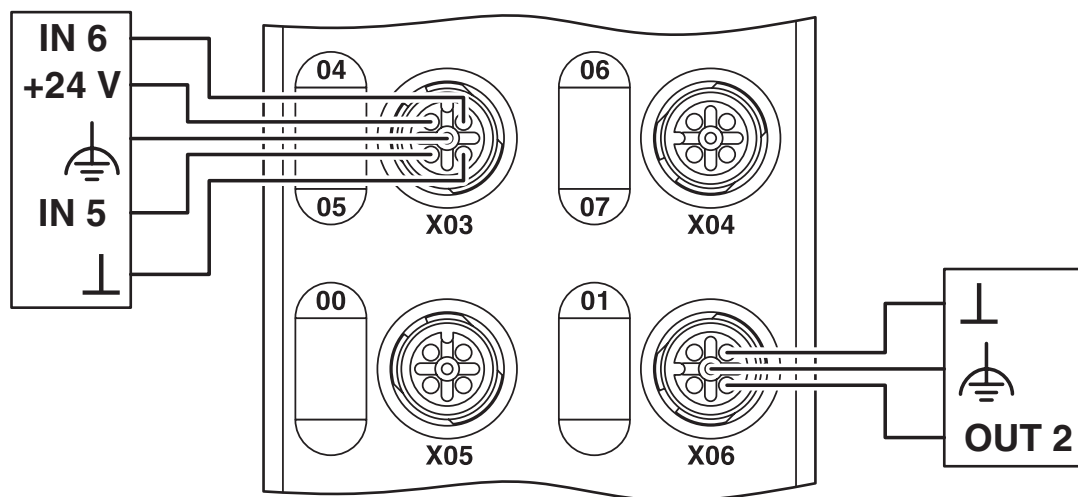
rysunek złączy
