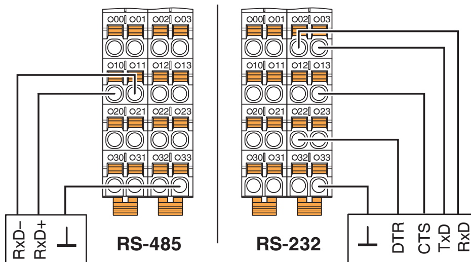
rysunek złączy
