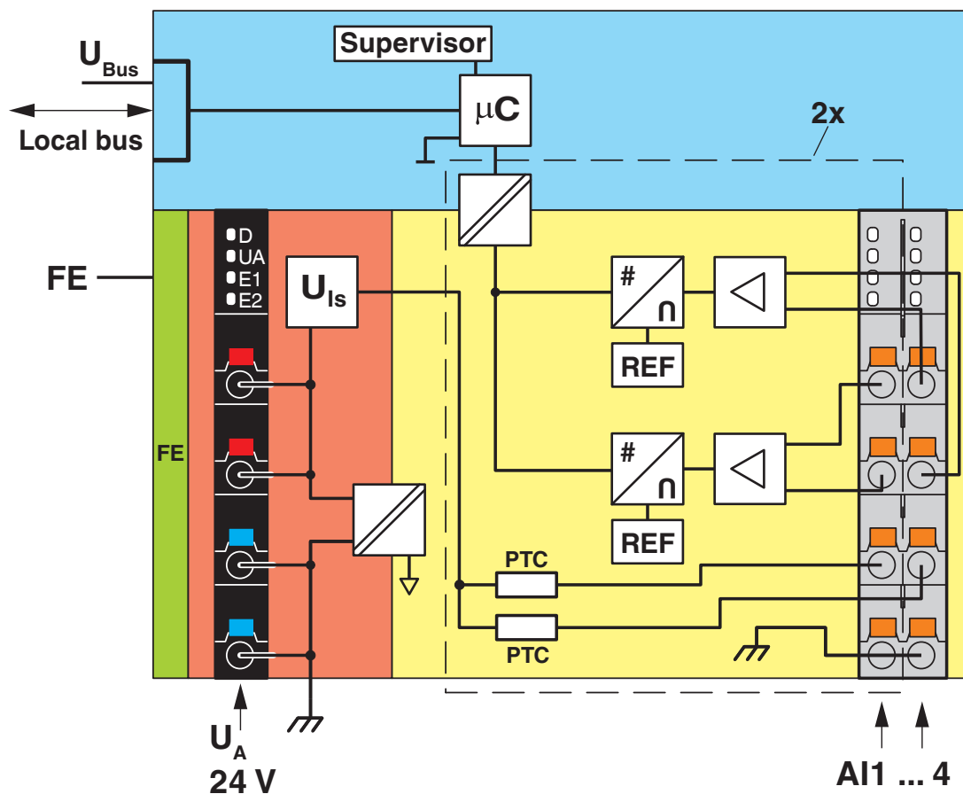
Schemat blokowy
