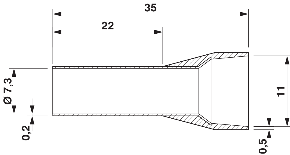
Rysunek wymiarowy
