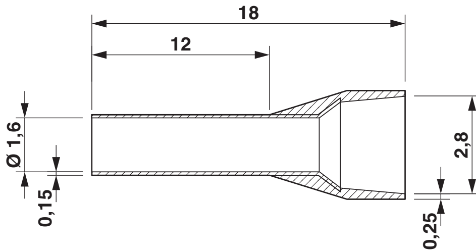
Rysunek wymiarowy
