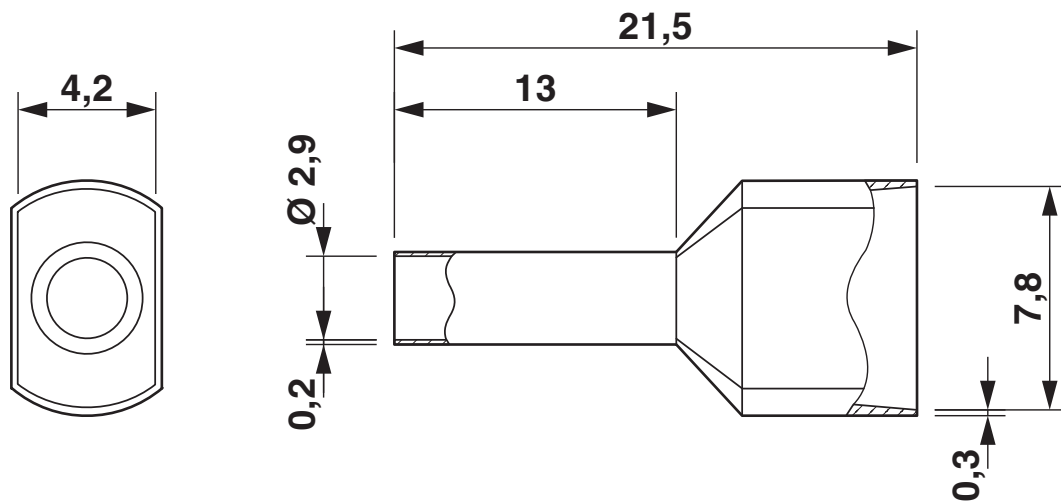
Rysunek wymiarowy
