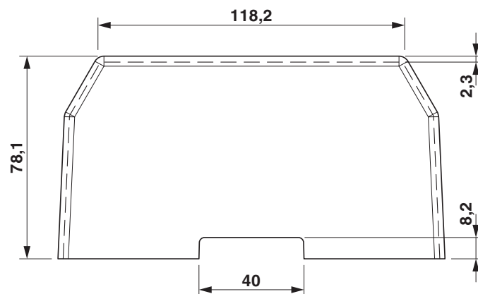
Rysunek wymiarowy
