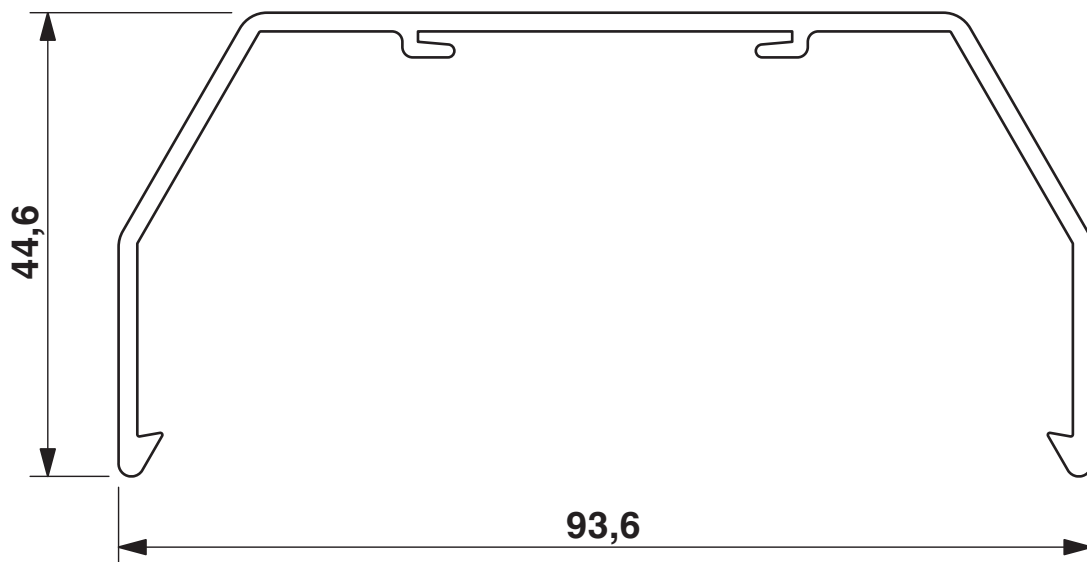
Rysunek wymiarowy
