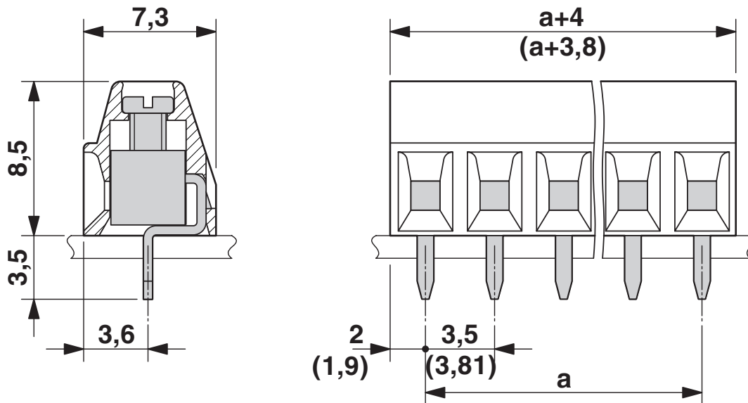
Rysunek wymiarowy
