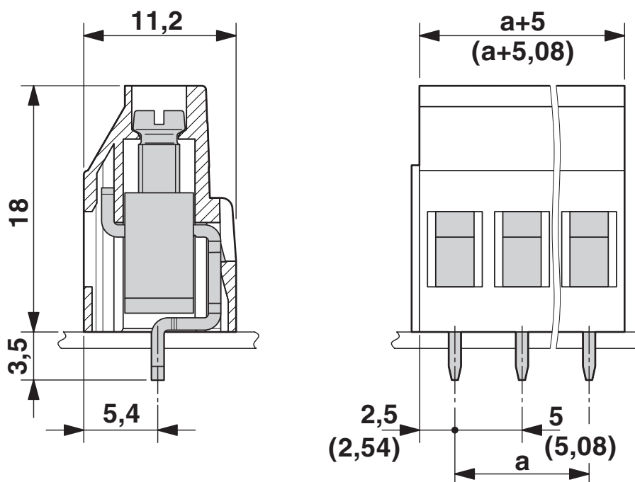
Rysunek wymiarowy
