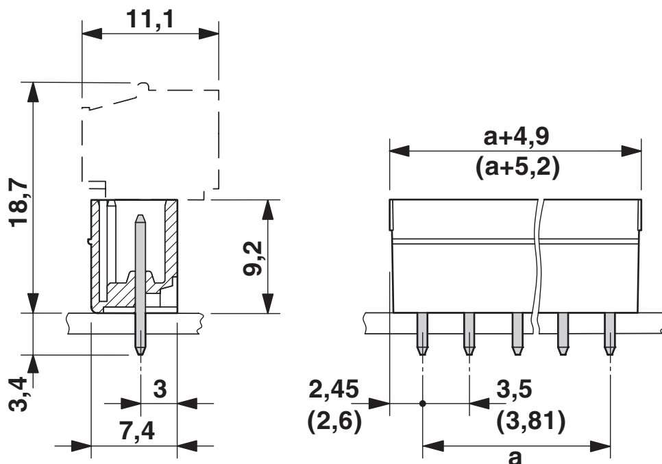
Rysunek wymiarowy
