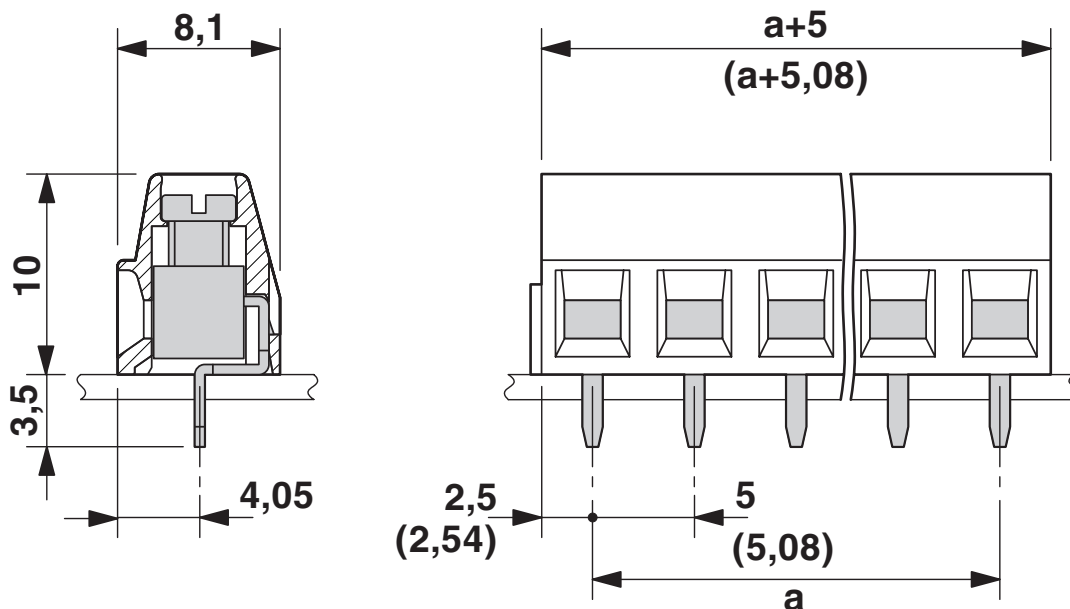
Rysunek wymiarowy
