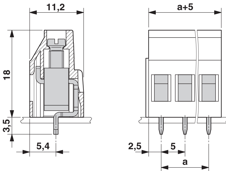
Rysunek wymiarowy
