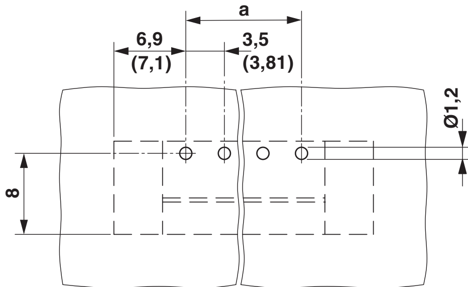
Rysunek wymiarowy
