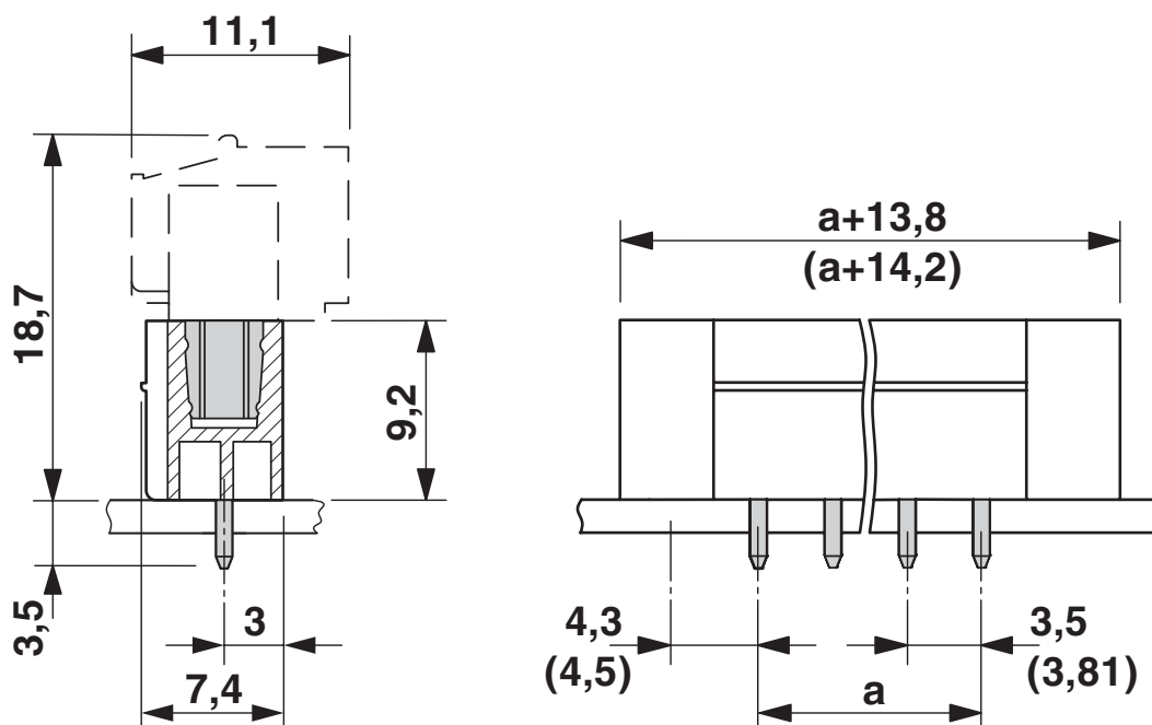
Rysunek wymiarowy
