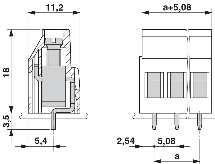
Rysunek wymiarowy
