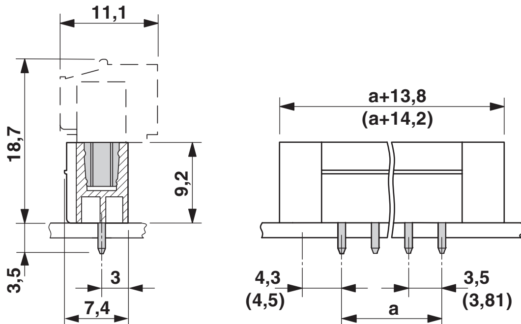
Rysunek wymiarowy
