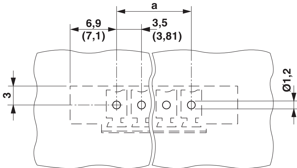
Rysunek wymiarowy
