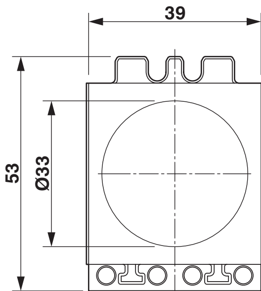
Rysunek wymiarowy
