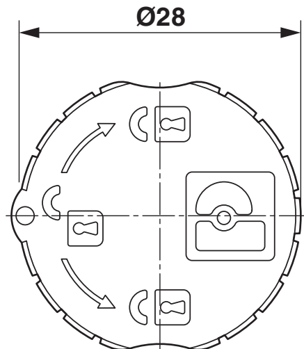
Rysunek wymiarowy
