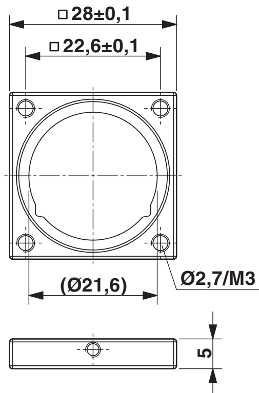
Rysunek wymiarowy
