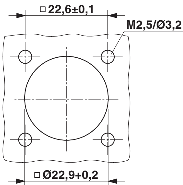
Rysunek wymiarowy
