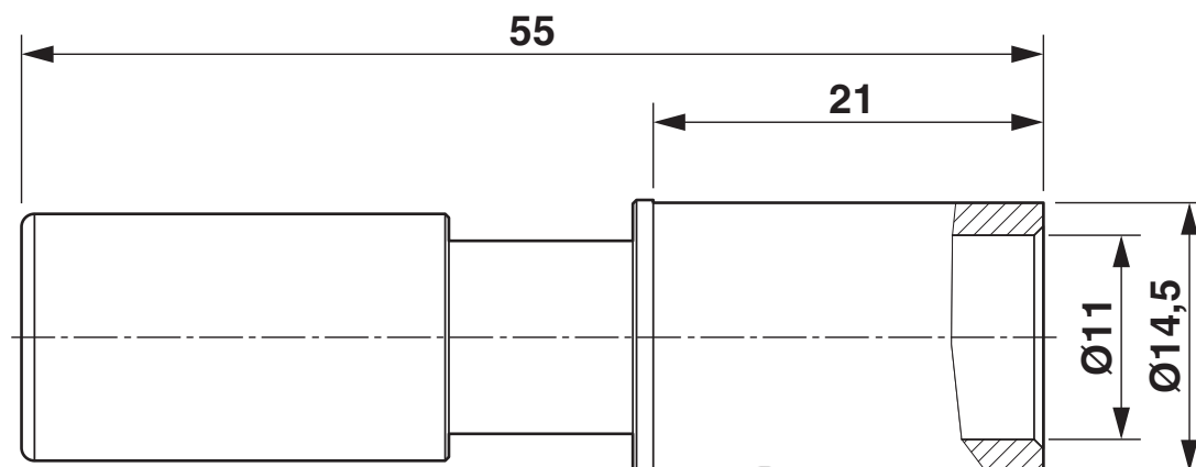
Rysunek wymiarowy
