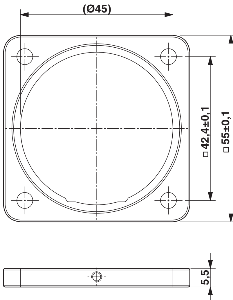
Rysunek wymiarowy
