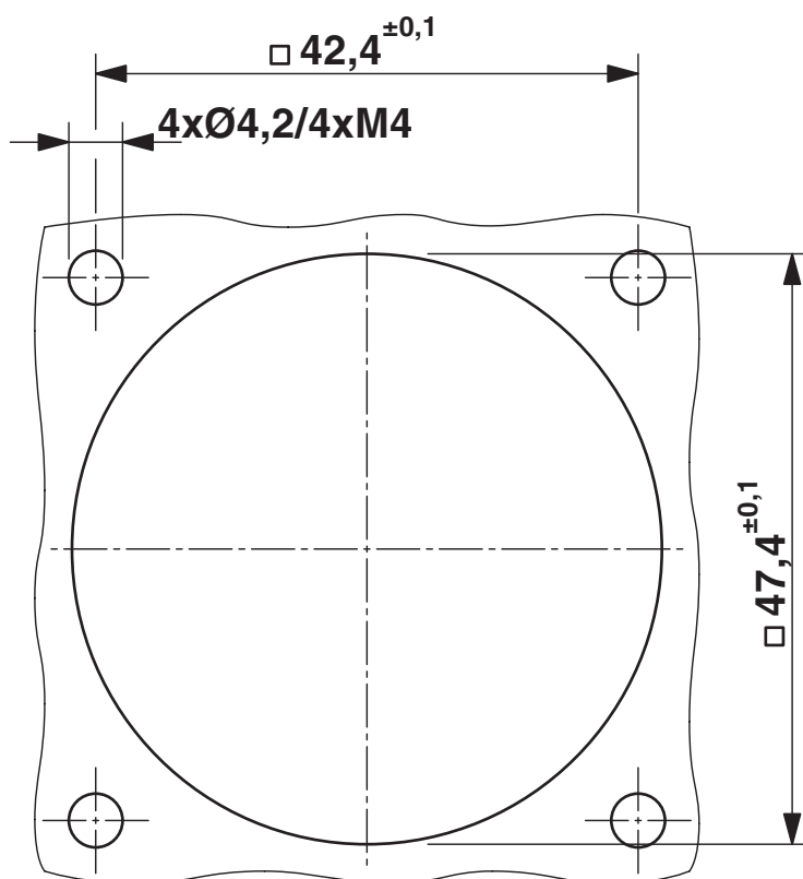
Rysunek wymiarowy
