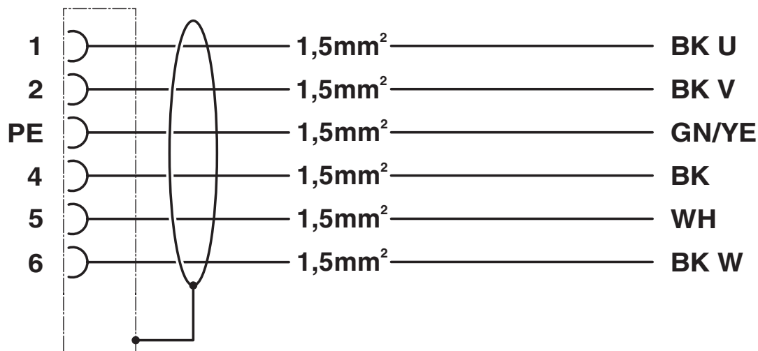
Schemat
