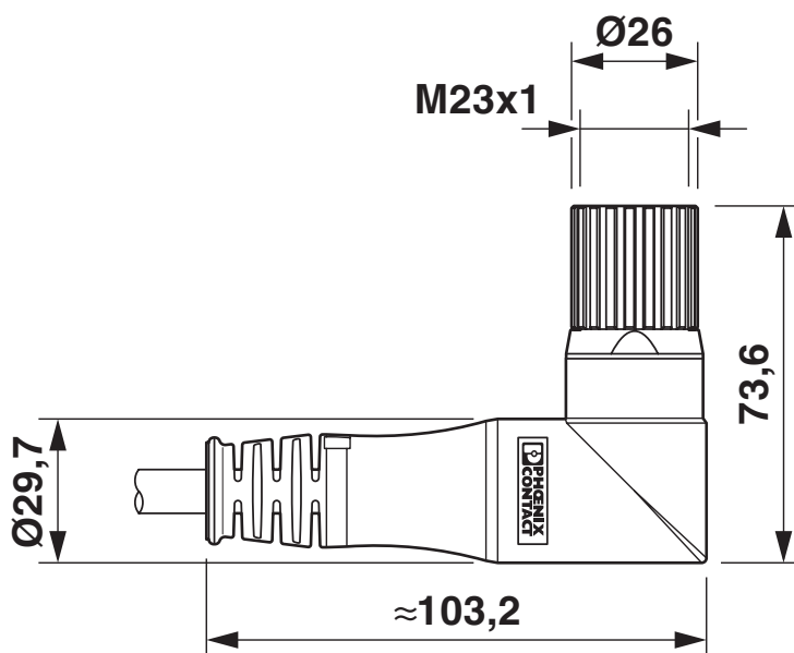
Rysunek wymiarowy
