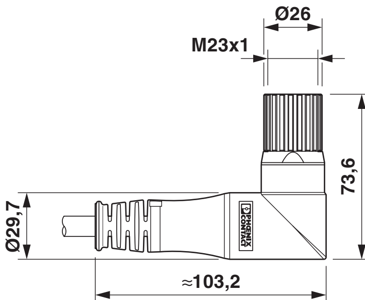
Rysunek wymiarowy
