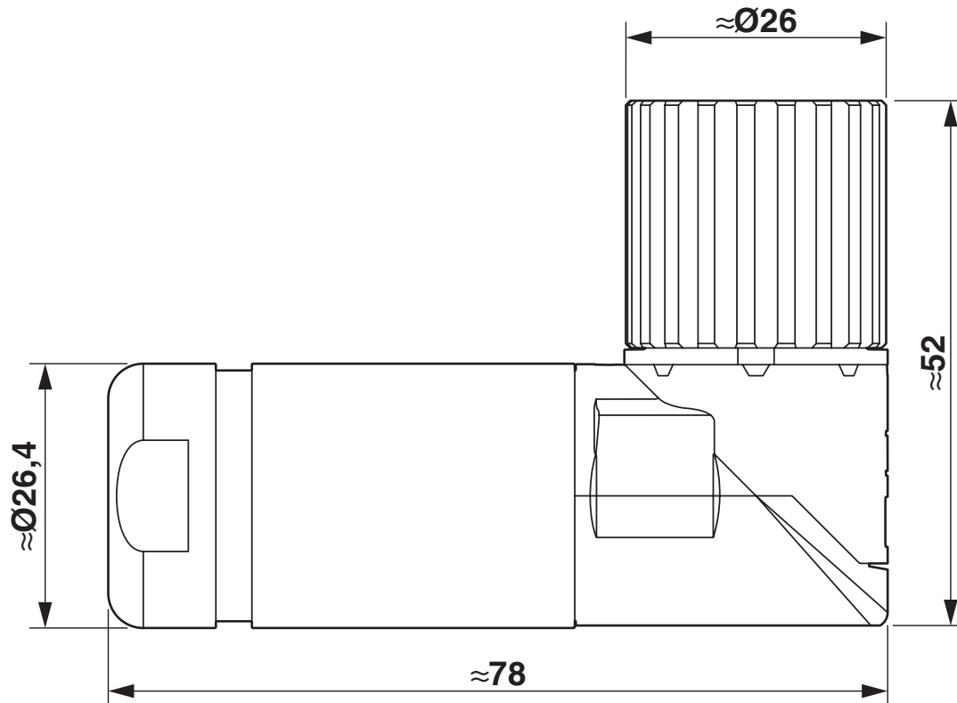
Rysunek wymiarowy
