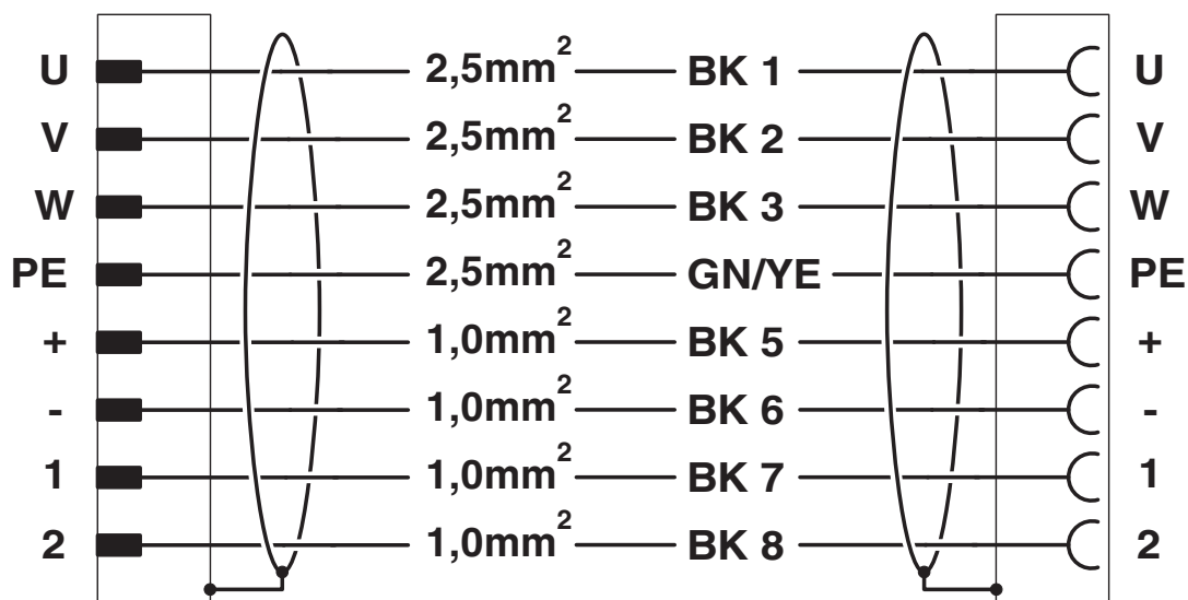
Schemat
