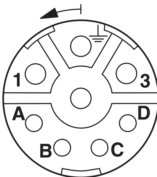
Rysunek schematyczny
