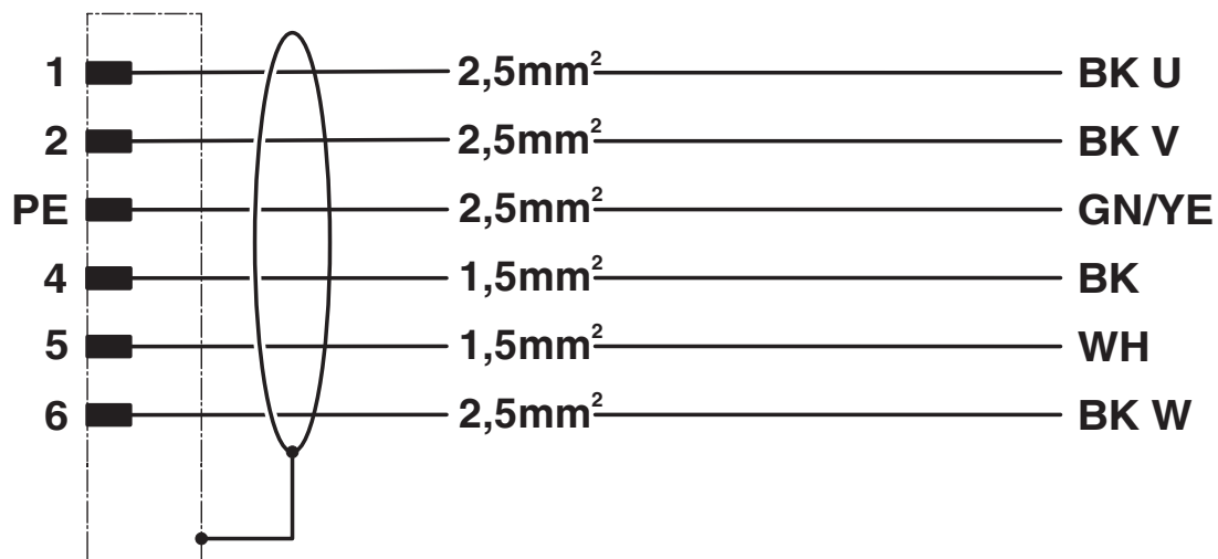
Schemat
